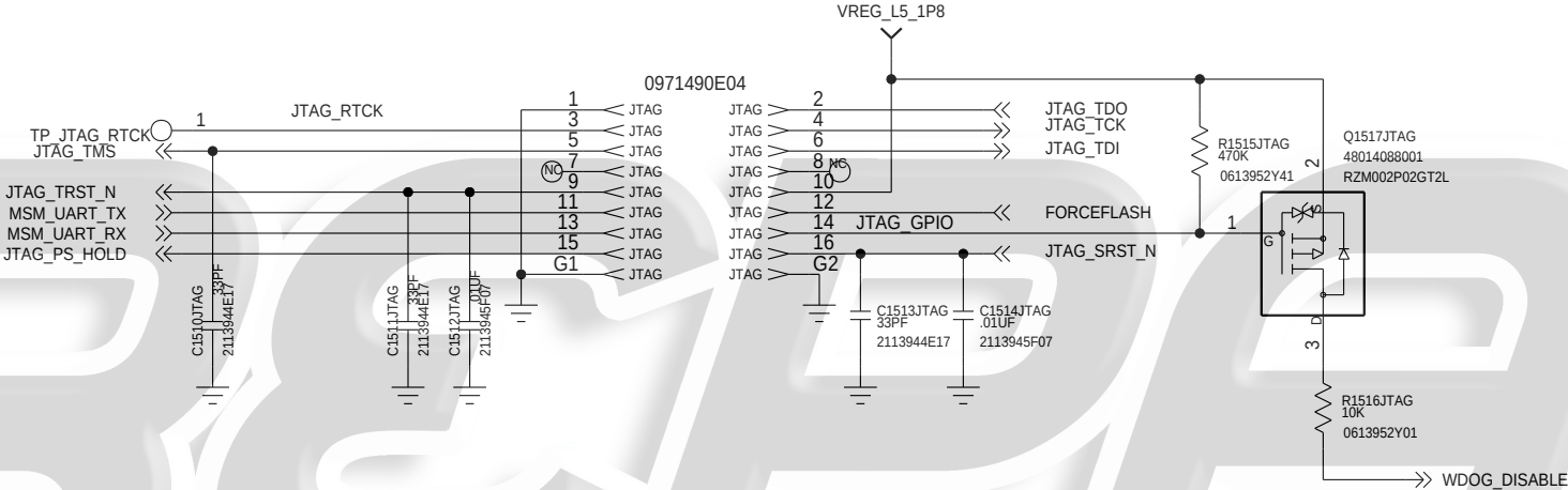
JTAG:MINI
